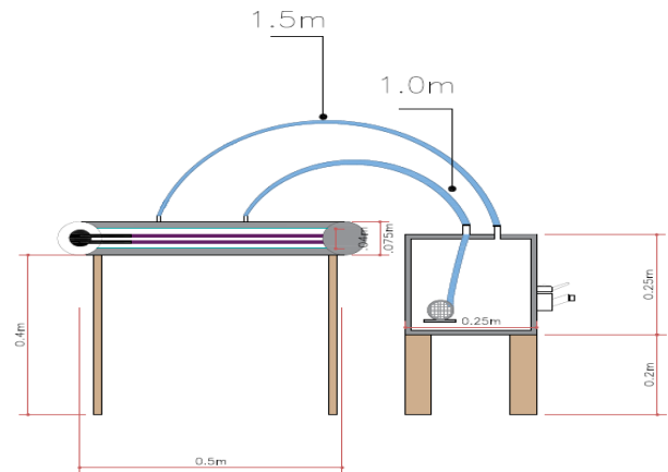
FIGURA 05: SISTEMA COM RESERVATÓRIO E FILTRO
